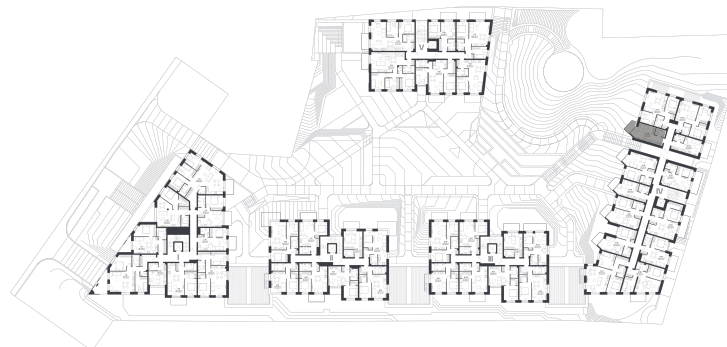
Patalpos aukšte
